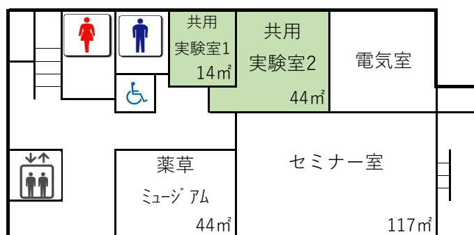
1階平面図
