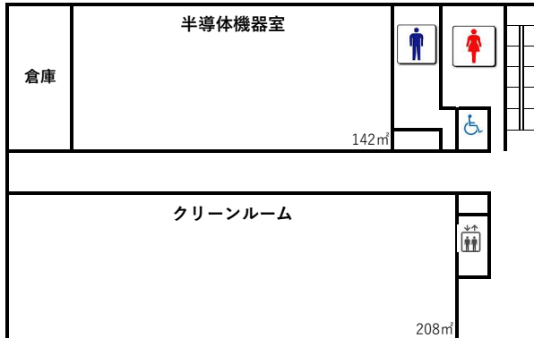
5階平面図
